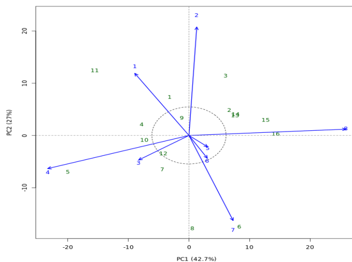
شکل ۴- بای پلات دو مؤلفه اصلی (PC2 و PC1) برهم کنش ژنوتیپ \times محیط در مدل 2 AMMI برای عملکرد ۱۶ ژنوتیپ عدس در محیط ۸
