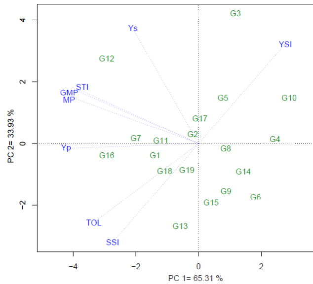
شکل ۳- بای پلات مبتنی بر دو مولفه اول حاصل از تجزیه به مؤلفه‌های اصلی براساس مقادیر عملکرد دانه در شرایط تنش و بدون تنش و شاخص‌های مقاومت به خشکی برآورد شده برای ۱۹ ژنوتیپ مورد بررسی
