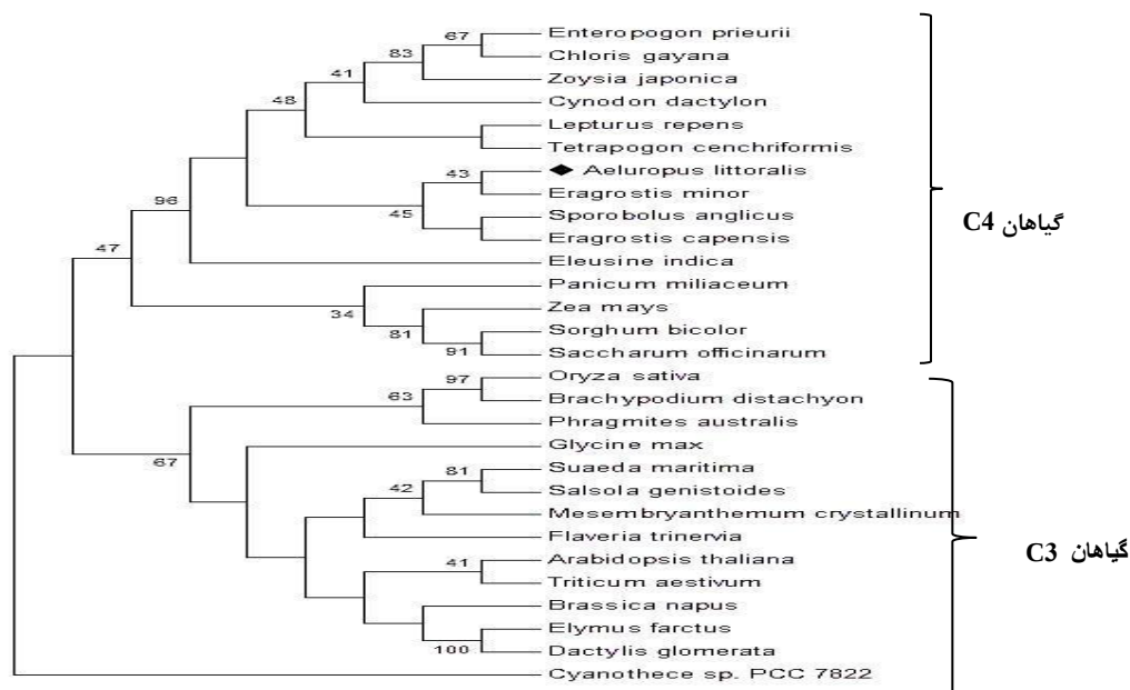
شکل ۲- مقایسه قرابت توالی پروتئینی PEPC آلورپوس لیترالیس و سایر گونه‌ها. درخت فیلوژنتیکی با استفاده از نرم‌افزار MEGA4 و روش اتصال مجاور (neighborjoining) ترسیم شد. و پارامتر تکرار در ترسیم ۱۰۰۰ در نظر گرفته شد.
