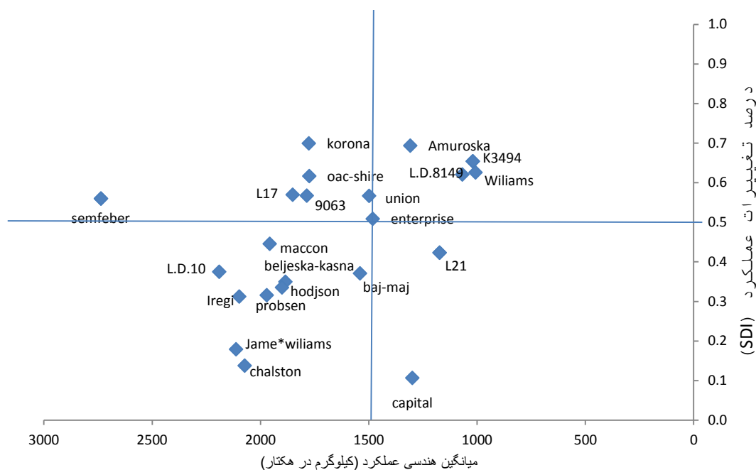
نمودار ۱- مقایسه ژنوتیپ‌ها از نظر دو شاخص میانگین هندسی و درصد تغییرات عملکرد Chart 1. Compare of genotypes by GMP and SDI indices
