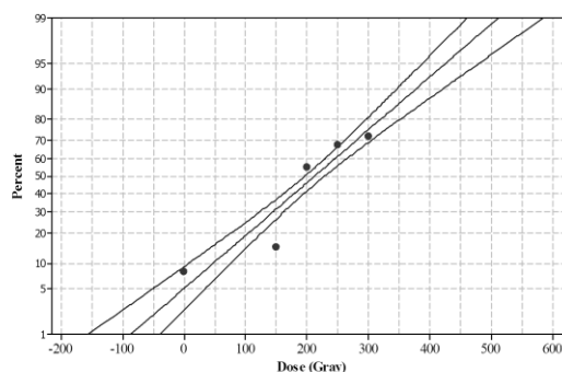
شکل ۱- تجزیه پروبیت برای تعیین دز ۵۰٪ کشته در هیبرید سینگل کراس ۷۰۴ Figure 1. Probit analysis for LD50 determination in hybrid SC704
