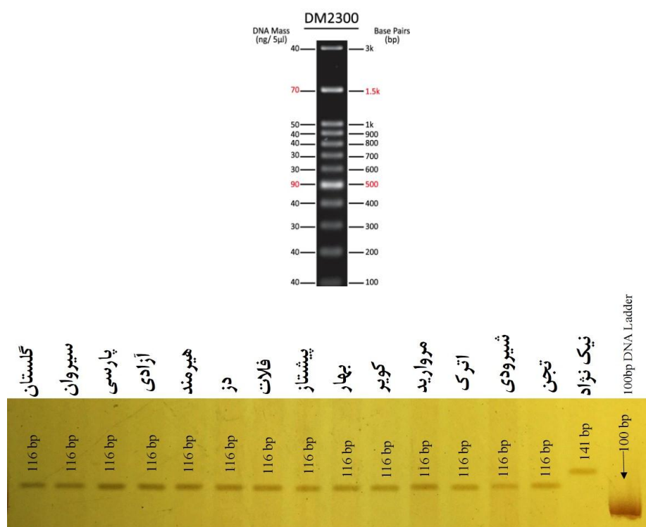
شکل ۳- الگوی باندی حاصل از تکثیر توسط آغازگر 22 /7D (اندازه نوارها تقریبی است) و Excel Band 100 bp DNA Ladder Figure 3. Banding pattern of the amplified using 22 /7D primer (Band sizes are approximate) and Excel Band 100 bp DNA Ladder
