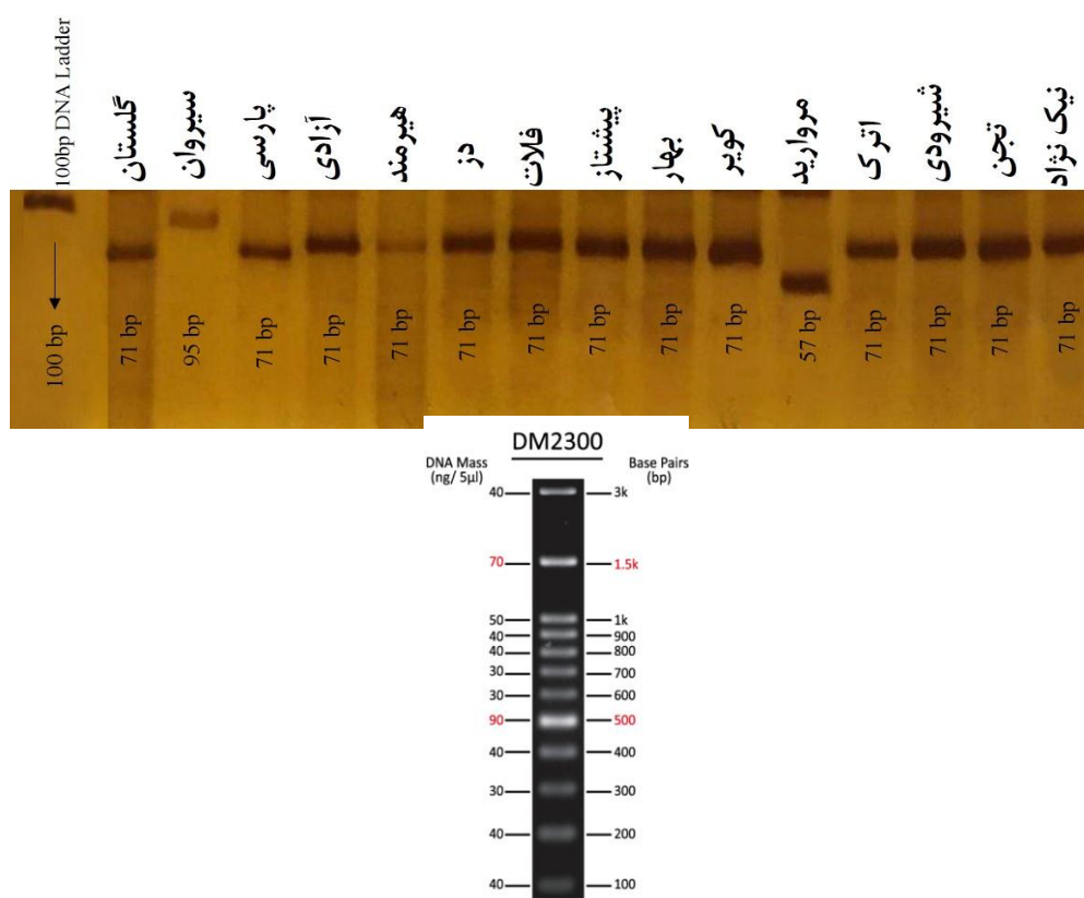
شکل ۴- الگوی بانندی حاصل از تکثیر توسط آغازگر 25 /5B (اندازه نوارها تقریبی است) و Excel Band 100 bp DNA Ladder
