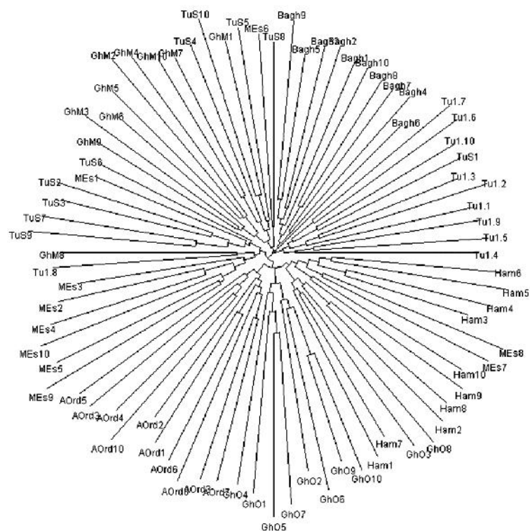
شکل ۱- دندروگرام افراد یونجه مورد مطالعه به روش Neighbor Joining بر اساس ۳۶۹ نشانگر IRAP, REMAP, ISSR و SSR (GhM): قره یونجه ملک کندی، GhO: قره یونجه ارومیه، MES: محلی اصفهان، Bagh: بغدادی، Ham: همدانی، Aord: آذربایجان اردوباد، Tu: الچی، TuS: ساکول
