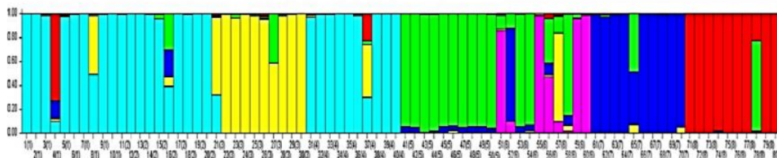
شکل ۲- تجزیه کلاستر مبتنی بر مدل Bayesian برای ۸۰ فرد یونجه بر اساس ۳۶۹ نشانگر IRAP، REMAP، ISSR و SSR ( K=6 ). هر رنگ یک زیر جمعیت یا کلاستر را نشان می‌دهد. اعداد روی محور افقی و عمودی به ترتیب شماره افراد و ضریب تعلق هر فرد به هر کلاستر را نشان می‌دهد.
