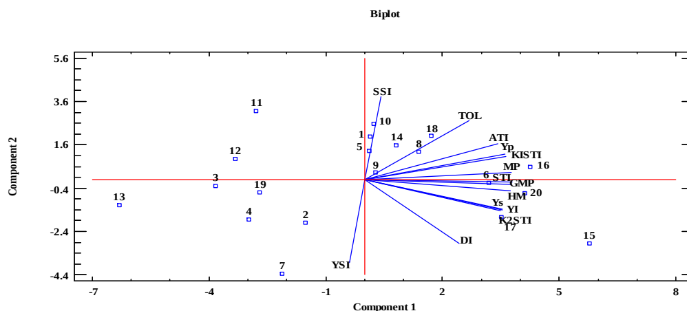
شکل ۳- نمودار بای پلات دو مولفه اول تجزیه به مولفه‌های اصلی در آزمایش تنش خشکی بعد از آبستنی که در آن موقعیت شاخص‌ها و ارقام مورد مطالعه مشخص شده است. شماره‌های ۱ تا ۲۰ روی نمودار بای پلات به ترتیب مربوط به ارقام زیر می‌باشد:
