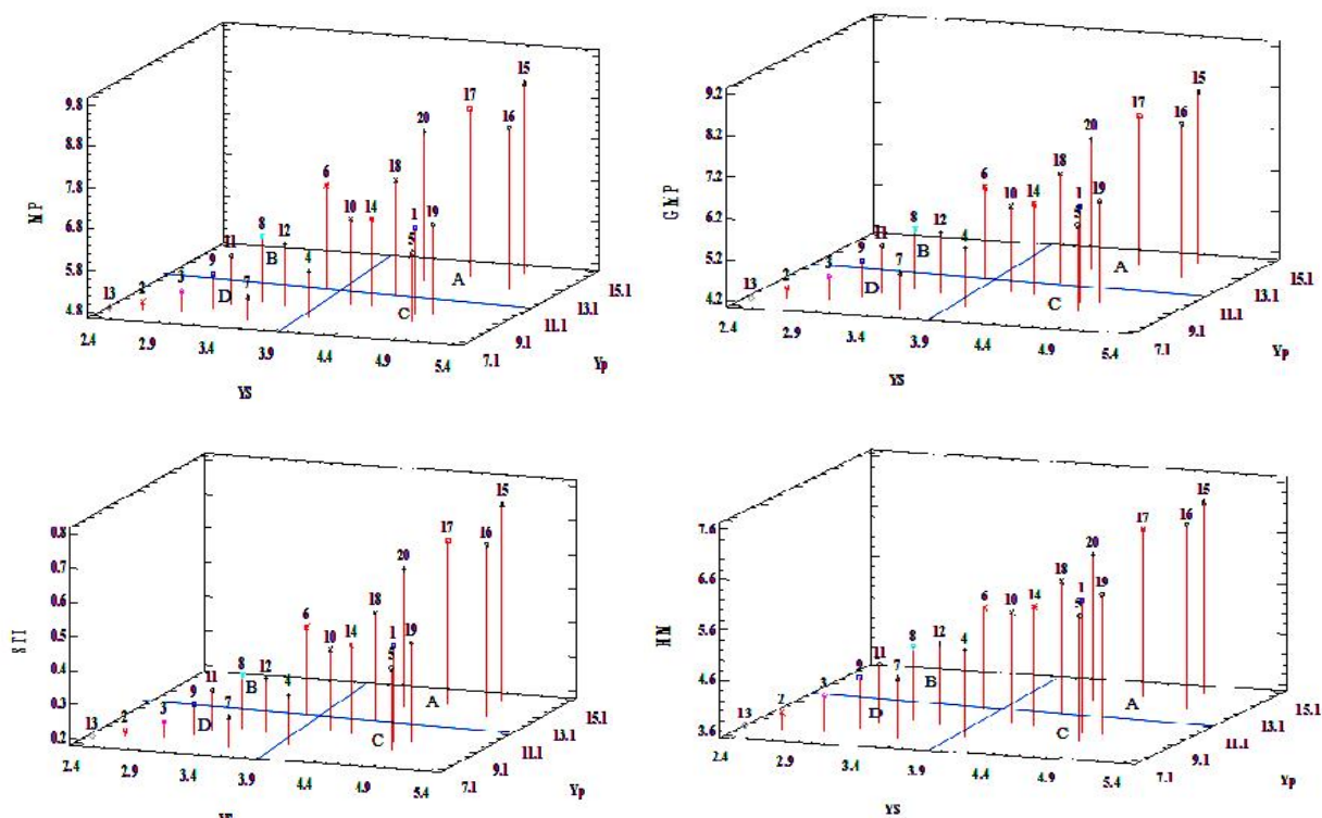
شکل ۲- نمودار سه بعدی عملکرد دانه (بر حسب گرم در بوته) در شرایط آبیاری کامل (Yp) و عملکرد دانه (بر حسب گرم در بوته) در شرایط تنش خشکی قبل از آبستنی (YS) با شاخص‌های MP, GMP, STI و HM.
