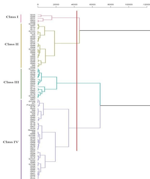
شکل ۲- تجزیه خوشه‌ای ژنوتیپ‌های مختلف جو براساس ضریب فاصله اقلیدوسی و الگوریتم خوشه‌بندی Ward Figure 2. Cluster analysis of different barley genotypes based on the Euclidean distance coefficient and Ward's clustering algorithm
