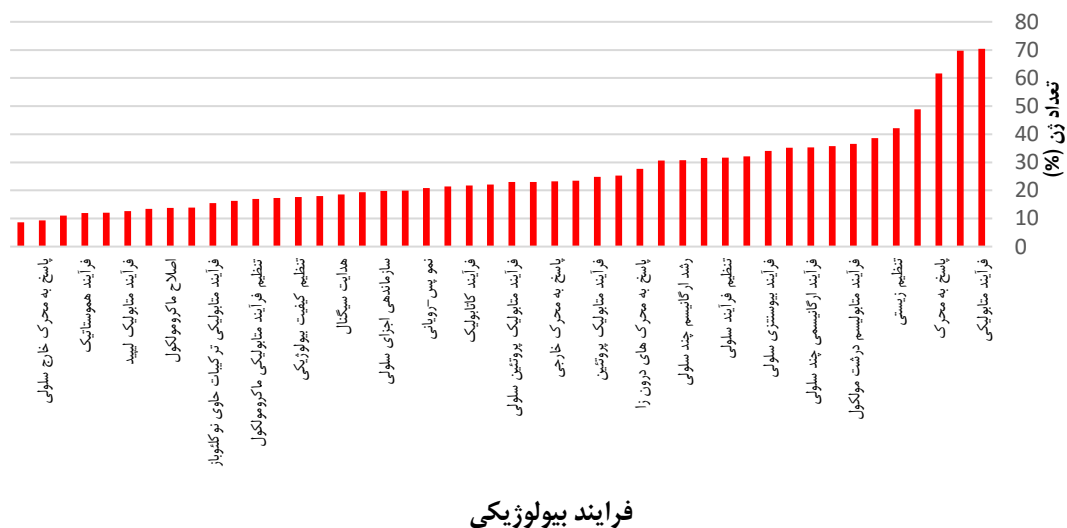
شکل ۳- هستی‌شناسی ژن‌های دارای بیان افتراقی تحت تنش خشکی انتهایی فصل براساس فرایندهای بیولوژیک Figure 3. Ontologies of differentially expressed genes under terminal drought stress based on biological processes
