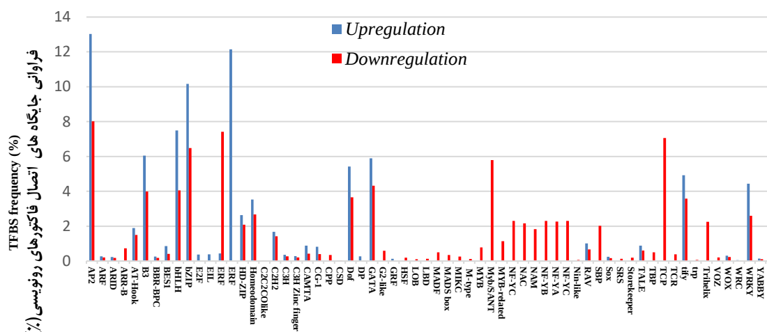
شکل ۱- جایگاه‌های اتصال عوامل رونویسی در ژن‌های شناسایی شده تحت تنش خشکی انتهای فصل Figure 1. Transcription factor binding sites in genes indentified under termainal drought stress
