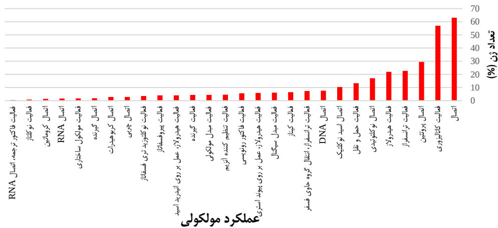
شکل ۲- هستی‌شناسی ژن‌های دارای بیان افتراقی تحت تنش خشکی انتهای فصل براساس عملکرد مولکولی
