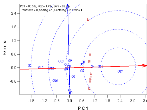
شکل ۵- نمایش بای‌پلات ژنوتیپ \times عملکرد \times صفت برای مقایسه ژنوتیپ‌های مورد مطالعه با ژنوتیپ ایده‌آل در کلزا Figure 5. The view of the genotype \times yield \times trait biplot to compare the studied genotypes with the ideal genotype in rapeseed
