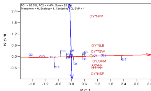
شکل ۶- مختصات تستر متوسط (ATC) بای‌پلات ژنوتیپ \times عملکرد \times صفت جهت رتبه‌بندی ژنوتیپ‌ها بر اساس برتری کلی و تعیین نقاط قوت و ضعف آن‌ها. DF: روز تا گلدهی، DPM: روز تا رسیدگی فیزیولوژیک، PH: ارتفاع بوته، NLB: تعداد شاخه فرعی، NPP: تعداد غلاف در بوته، NSP: تعداد دانه در غلاف، TSW: وزن هزاردانه، OC: درصد روغن، OY: عملکرد روغن
