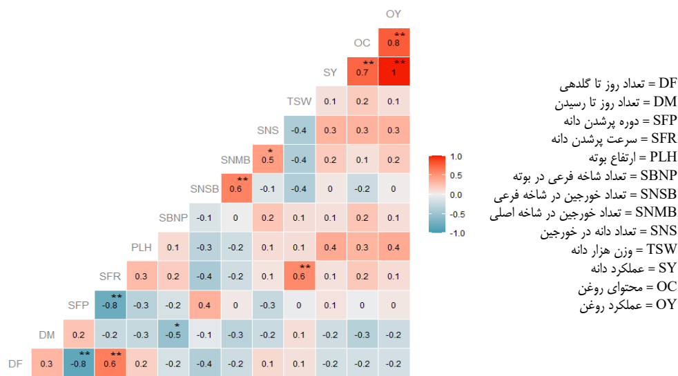
شکل ۱- نقشه دمایی به دست آمده بر اساس ضرایب همبستگی پیرسون Figure 1. Heat map rendered based on Pearson's correlation coefficients
