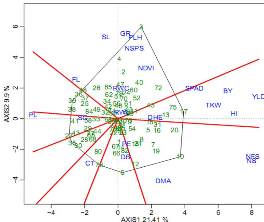
شکل ۳- بای پلات چندضلعی ژنوتیپ در صفت برای ۸۸ ژنوتیپ گندم دوروم بر اساس ۲۲ صفت مورد بررسی در شرایط دیم Figure 3. Polygon view of GT biplot for 86 durum wheat genotypes based on 22 studied traits under rainfed condition
