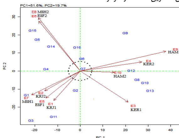
شکل ۲ - نمودار بایپلات بر اساس دو مؤلفه اصلی اول اثر متقابل (AMMI2) Figure 2. Biplot based on value of tow main principal components of interaction (AMMI2)
