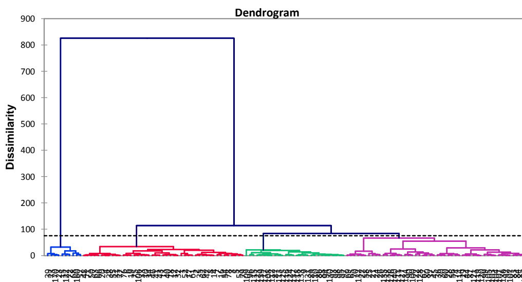
شکل ۲- گروه‌بندی خوشه‌ای ژنوتیپ‌های ارزن دم‌روبه‌ای Figure 2. Cluster analysis-based dendrogram of investigated traits of foxtail millet genotypes
