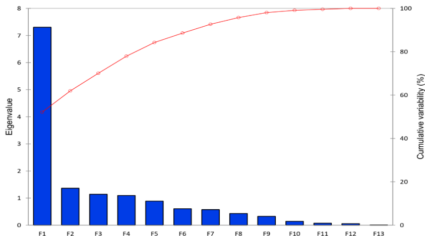
شکل ۱- اسکرین پلات مقادیر هر یک از مؤلفه‌های اصلی صفات فنوتیپی مجموعه ژرم پلاسما ارزن دم‌روبه‌ای Figure 1. The principal screen plot of foxtail millet germplasm
