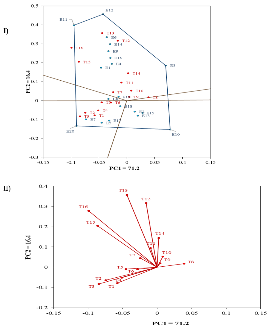
شکل ۲- I) نمودار بای پلات ۲۰ اکوتیپ گاو دانه و ۱۶ صفت مورفولوژیکی و فنولوژیکی و II) بای پلات ۱۶ صفت مورفولوژیکی و فنولوژیکی (کد و نام اکوتیپ های گاو دانه و صفات مورد مطالعه به ترتیب در جداول ۱ و ۴ ارائه شده است)
