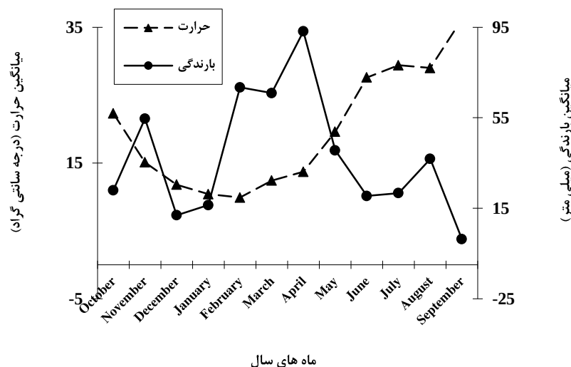
شکل ۲- آمار هواشناسی آمبروترمیک کوتاه مدت ایستگاه هواشناسی سینوپتیک گنبد کاووس (۱۳۹۸-۱۳۹۹)
