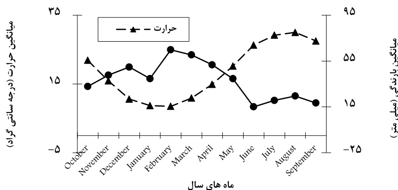
شکل ۱- آمار هواشناسی آمبروترمیک بلندمدت ایستگاه هواشناسی سینوپتیک گنبد کاووس (۱۳۷۱-۱۳۹۸)
