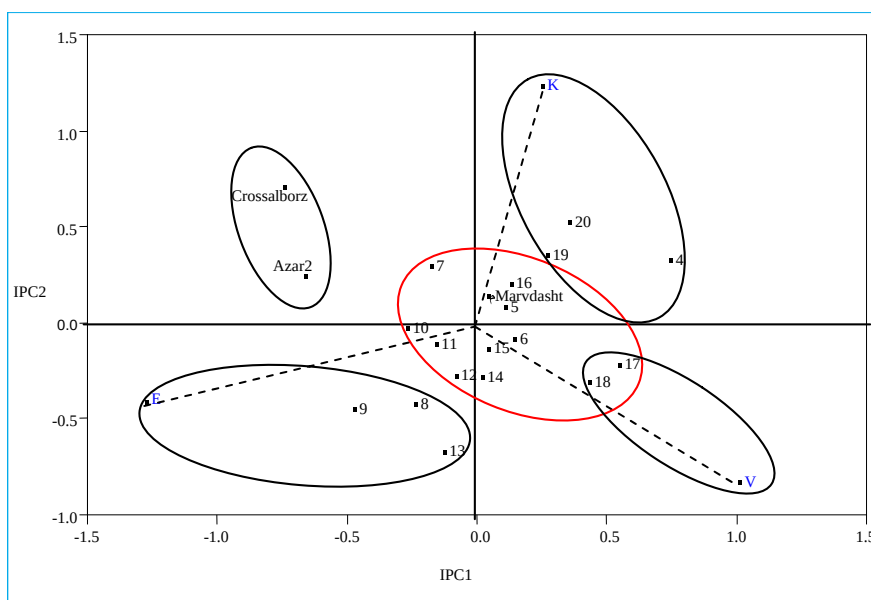
شکل ۳- بای پلات حاصل از میانگین و پایداری IPC1 و IPC2 ژنوتیپ‌ها و محیط‌ها.
