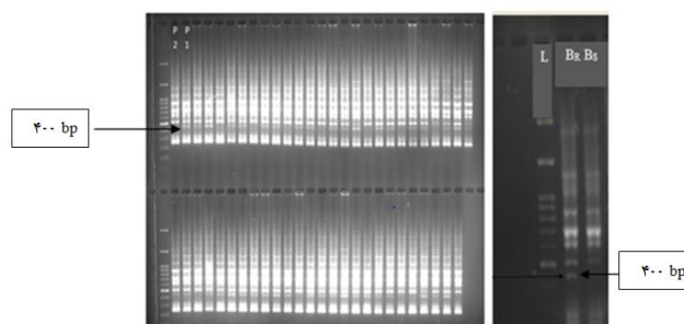
شکل ۲- الگوی چندشکلی نشانگر ISSR-5 در افراد جمعیت F_2 تلاقی 1528 \times 164 , P_1 (والد مقاوم)، P_2 (والد حساس)، B_R (بالک مقاوم) و B_S (بالک حساس)، L : نشانگر وزنی ۱۰۰ bp Figure 2. Polymorphism pattern of the ISSR-5 primer in F_2 populations of 1528 \times 164 , P_1 (resistant parent), P_2 (susceptible) size marker (100 bp)
