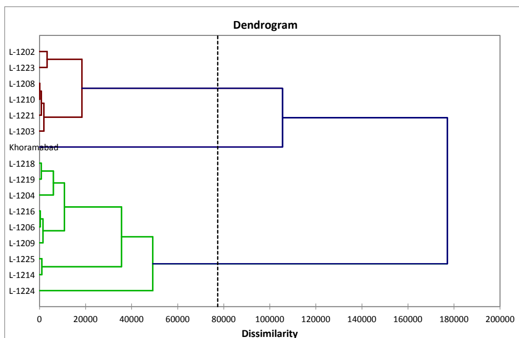
شکل ۱- نمودار درختی حاصل از تجزیه خوشه‌ای براساس شاخص‌های تحمل به خشکی در شرایط نرمال و تنش خشکی Figure 1. Dendrogram obtained from cluster analysis based on tolerance indices in normal and drought stress conditions
