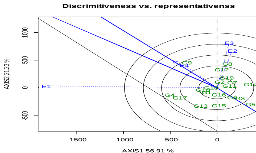
شکل ۶- نمای قدرت تمایز و نمایندگی محیط‌ها یا مقیاس بندی مبتنی بر محیط ۱ و PC2، به‌ترتیب مولفه اصلی اول و دوم هستند 6. View of the power of differentiation and representation of environments or scaling based on environment. Fig PC1 and PC2 are the first and second principal components, respectively
