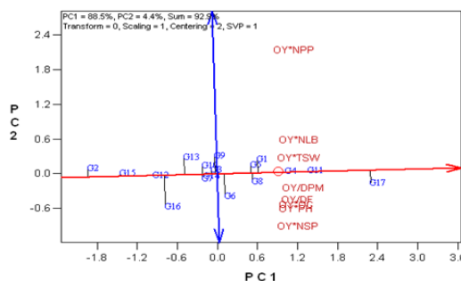
شکل ۶- مختصات تستر متوسط (ATC) بای‌پلات ژنوتیپ × عملکرد × صفت جهت رتبه‌بندی ژنوتیپ‌ها بر اساس برتری کلی و تعیین نقاط قوت و ضعف آن‌ها. DF: روز تا رسیدگی فیزیولوژیک، PH: ارتفاع بوته، NLB: تعداد شاخه فرعی، NPP: تعداد غلاف در بوته، NSP: تعداد دانه در غلاف، TSW: وزن هزاردانه، OC: درصد روغن، OY: عملکرد روغن
