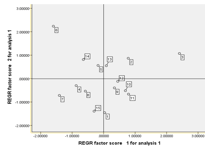
شکل ۱- گروه‌بندی ژنوتیپ‌های مطالعه شده با استفاده از شاخص‌های محاسبه شده از طریق تجزیه به مؤلفه‌های اصلی Figure 1. Grouping of studied genotypes using calculated indices through principal component analysis
