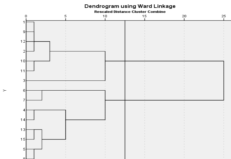
شکل ۲- گروه‌بندی ژنوتیپ‌های مطالعه شده با استفاده از شاخص‌های محاسبه‌شده از طریق تجزیه خوشه‌ای Figure 2. Grouping of studied genotypes using calculated indices through cluster analysis
