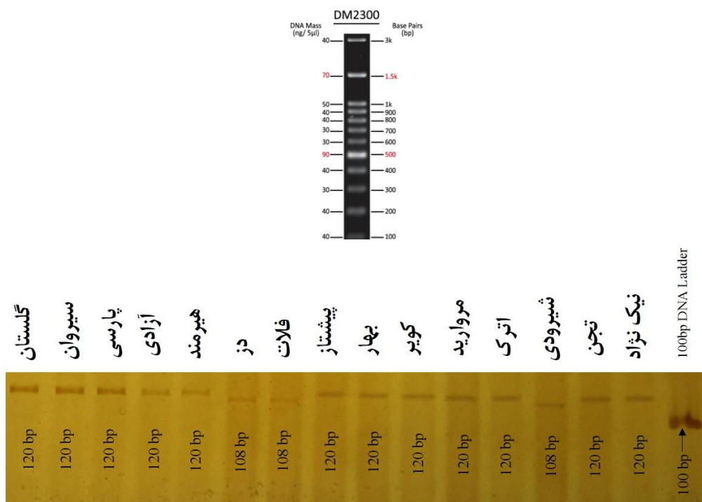
شکل ۱- الگوی باندی حاصل از تکثیر توسط آغازگر 15/2A (اندازه نوارها تقریبی است) و Excel Band 100 bp DNA Ladder Figure 1. Banding pattern of the amplified using 15/2A primer (Band sizes are approximate) and Excel Band 100 bp DNA Ladder
