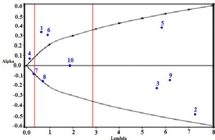
شکل ۲- نمودار برآورد شده با استفاده از رگرسیون تای، برای ارقام آفتابگردان مورد مطالعه (هذلولی فاصله برآورد ۹۵ درصد را برای =۰ نشان می‌دهد، خطوط عمودی حدود فاصله اطمینان ۹۵ درصد را برای =۱ نشان می‌دهد).
