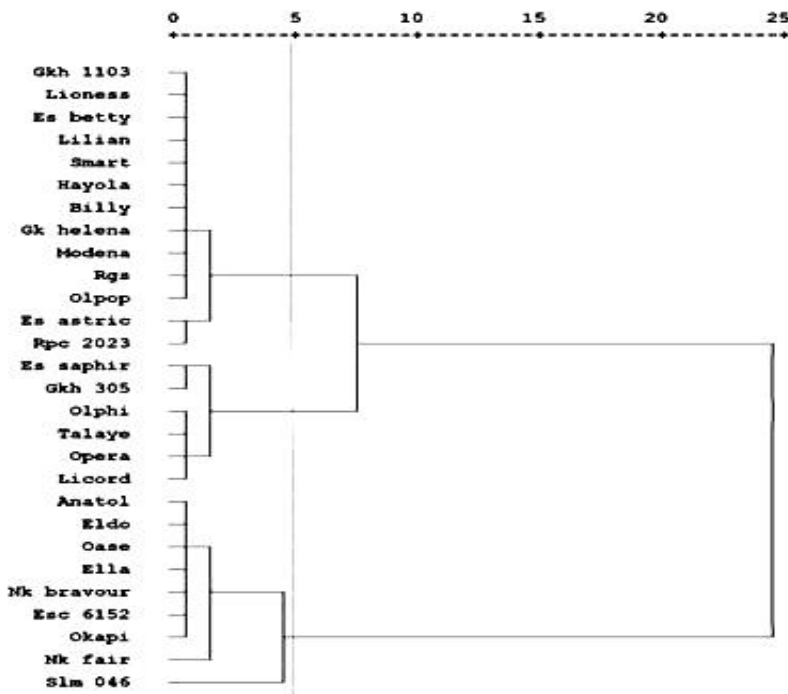
شکل ۲- نمودار خوشه‌ای به روش UPGMA ارقام مختلف کلزا بر اساس صفات مختلف مورد مطالعه در شرایط تنش رطوبتی.
