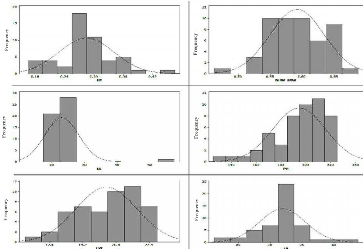
شکل ۱- توزیع فراوانی صفات مورفولوژیکی در توده‌های آفتابگردان آجیلی. محور عمودی نشان‌دهنده فراوانی هر دسته و محور افقی گروه‌های دسته‌بندی هر صفت را نشان می‌دهد. HI: شاخص برداشت، DHW-SW: نسبت مغز به کل تک دانه، LL: طول پهنک برگ، PH: ارتفاع بوته، LW: عرض پهنک برگ، LN: تعداد کل برگ، 100SW: وزن صد دانه، APDW: وزن خشک بوته (وزن خشک اندام هوایی منهای وزن خشک دانه در طبق)، CD: قطر طبق، CW: وزن خشک طبق، DF: تاریخ گلدهی، DHW: وزن مغز تک دانه، PL: طول دمیرگ، SSW: وزن تک دانه، SL: طول دانه، SD: قطر ساقه، SW: عرض دانه، YIELD: وزن خشک دانه در طبق.
