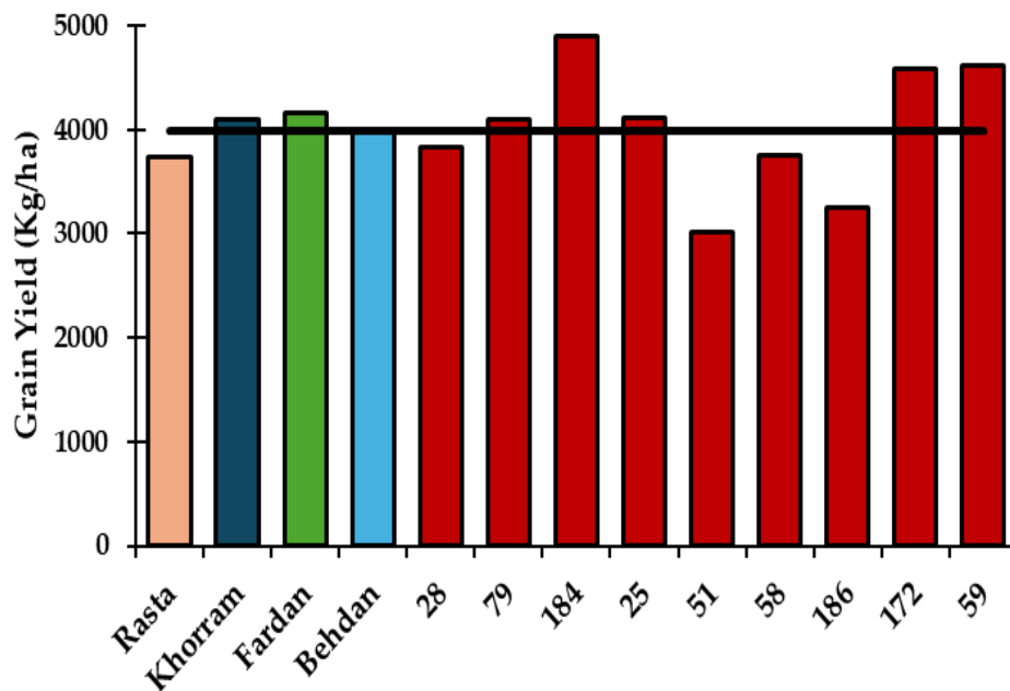
شکل ۵- مقایسه میانگین عملکرد نه ژنوتیپ برتر جو و چهار رقم شاهد (خط ممتد میانگین عملکرد چهار رقم شاهد را نشان می‌دهد). Figure 5. A comparison of average grain yields of the nine superior barley genotypes and four control cultivars (the solid line indicates the average yield of the four control cultivars)
