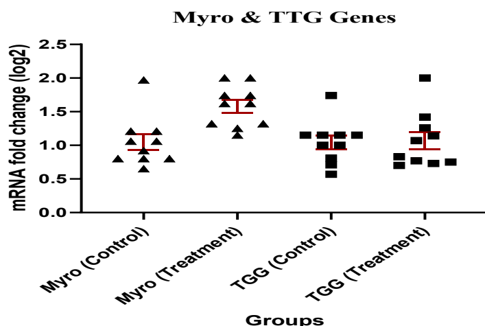
شکل ۴- نمودار مقایسه میزان تغییرات بیان ژن‌های میروزیناز و TTG در گیاه لگجی، (محور عمودی: میزان بیان نسبی، محور افقی: BMyro بیان نسبی برای ژن میروزیناز نمونه‌های محیط غیر رادیواکتیو، AMyro بیان نسبی برای ژن میروزیناز نمونه‌های محیط رادیواکتیو، BTTG بیان نسبی برای ژن BTTG نمونه‌های محیط غیر رادیواکتیو، ATTG بیان نسبی برای ژن TTG نمونه‌های محیط رادیواکتیو. Figure 4. mRNA fold change of Myrosinase (Myro) and TTG genes in C. ovata . (Y-axis represents the relative expression level. The X-axis represents four groups: BMyro (the control group for the myrosinase gene with none radon exposure), AMyro (the radon exposure group for the myrosinase gene), BTTG (the control group for the TTG gene), ATTG (the radon exposure group for the TTG gene).
