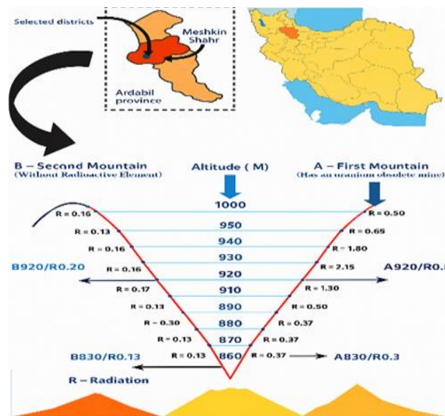
شکل ۱- نقشه شماتیکی نقاط نمونه برداری، ارتفاع و شدت تشعشعات رادیواکتیو در دو کوه مجاور هم (کوه اول (A) با تشعشعات رادیواکتیو بالا و کوه دوم (B، شاهد) بدون تشعشعات رادیواکتیو).
