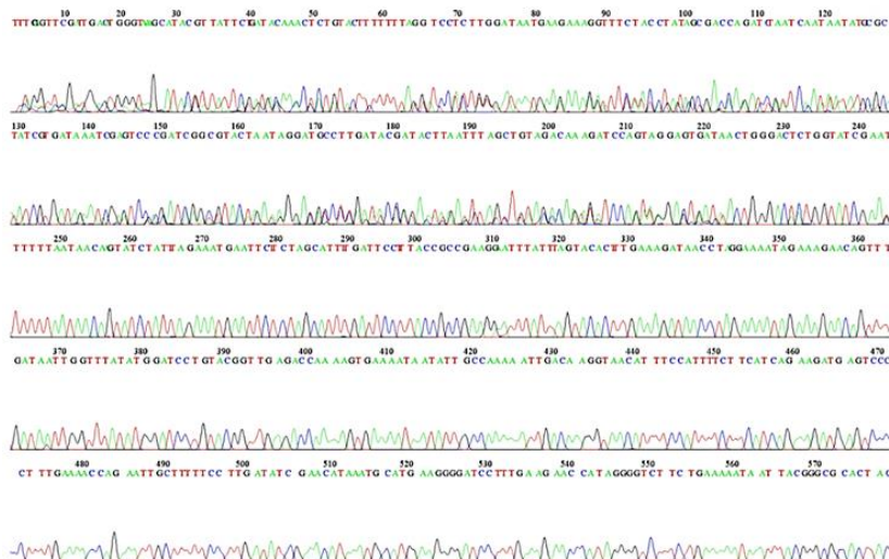
شکل ۲- گراف حاصل از نتایج توالی‌یابی ژن matK در خرماي سبزو به عنوان نمونه
