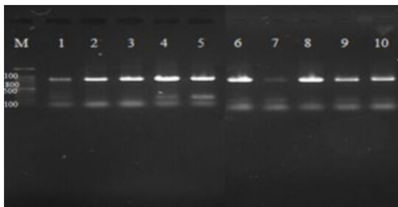
شکل ۱- محصولات PCR با آغازگرهای ژن matK برای ارقام ۱ تا ۱۰ خرماي مورد مطالعه.
