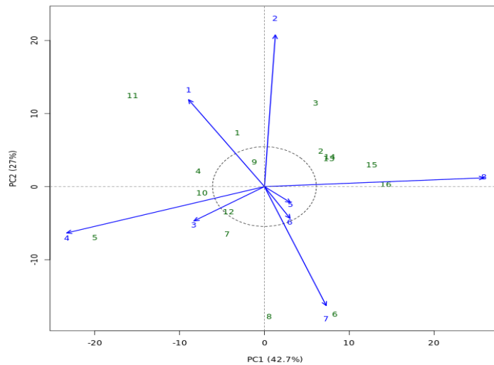
شکل ۴- بای پلات دو مؤلفه اصلی (PC1 و PC2) برهم کنش ژنوتیپ × محیط در مدل AMMI 2 برای عملکرد ۱۶ ژنوتیپ عدس در ۸ محیط
