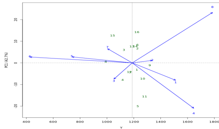
شکل ۳- بای پلات مؤلفه اصلی نخست (PC1) و عملکرد دانه (Y) (کیلوگرم در هکتار) در مدل AMMI 1 برای عملکرد ۱۶ ژنوتیپ عدس در محیط ۸
