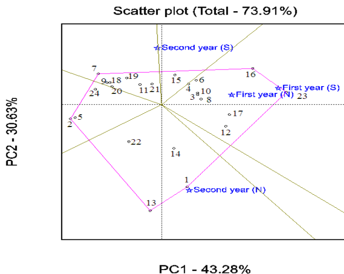
شکل ۱- نمای چندضلعی GGE بای پلات برای تعیین ژنوتیپ‌های برتر در محیط‌های مختلف، PC1= اولین مؤلفه اصلی، PC2= دومین مؤلفه اصلی
