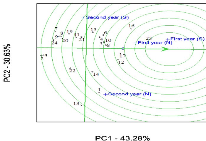
شکل ۲- نمودار GGE بای پلات بر اساس مقیاس‌بندی متمرکز شده روی ژنوتیپ‌ها برای مقایسه ژنوتیپ‌های ارزیابی شده با ژنوتیپ ایده‌آل در محیط ۶
