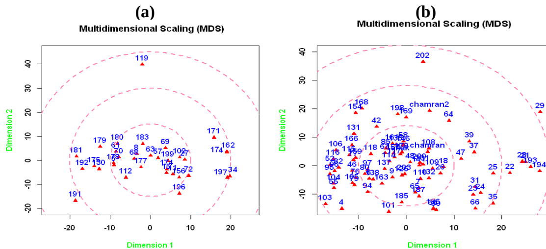
شکل ۴- تفکیک نمونه‌های ژنتیکی گروه اول (a) و گروه دوم (b) در تجزیه خوشه‌ای K means با استفاده از تجزیه مقیاس‌بندی چند بعدی در ارزیابی تحمل ژرم‌پلاسما گندم نان به تنش گرما در اهواز Figure 4. Distinction of the first group (a) and the second group (b) in K means clustering by Multi-dimensional scaling in tolerance evaluation of bread wheat germplasm to heat stress in Ahvaz
