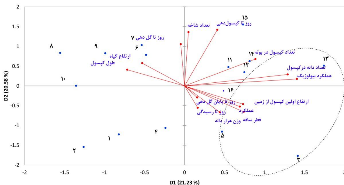
شکل ۱- بای‌پلات صفات کمی و پراکنش ژنوتیپ‌های کنگد مورد بررسی با استفاده از دو عامل اصلی حاصل از چرخش واریمکس Figure 1. Biplot of quantitative traits and evaluated sesame genotypes distribution using two first component of rotated varimax
