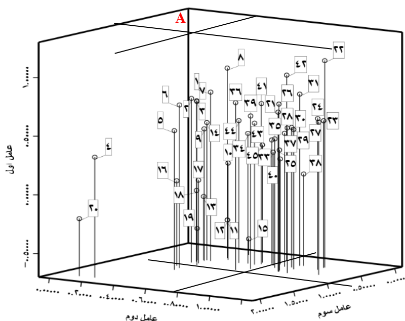
شکل ۳- نمودار سه بعدی پراکنش لاین‌های گندم دوروم بر اساس ضرایب عاملی (برای رسم نمودار پراکنش سه بعدی برای لاین‌ها، باید ضرایب مربوط به لاین‌ها برای هر تابع جداگانه مشخص شود. به این صورت که مجموع (تابع اول ضرب در صفت اول در لاین اول، تابع اول در صفت دوم در لاین اول) و به ترتیب برای تمام صفات در لاین ۱ تا ۴۵، همین کار را برای تابع دوم و سوم نیز انجام داده و عدد نهایی هر لاین را برای سه تابع را به صورت نمودار سه بعدی ترسیم می‌کنیم).
