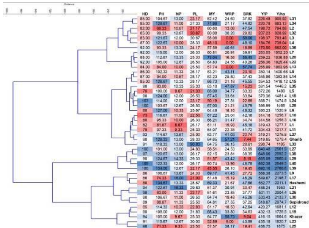
شکل ۲- گروه‌بندی ژنوتیپ‌ها بر اساس صفات مورفولوژیک به روش Ward در شرایط تنش خشکی. HD: تاریخ گلدهی، PH: ارتفاع بوته، NP: تعداد پنجه، PL: طول خوشه، MY: درصد کل تبدیل، WRP: درصد برنج سالم، BRK: درصد برنج خرد شده، Y/P: عملکرد در واحد پلات و Y/ha: عملکرد در واحد هکتار Figure 2. Grouping of genotypes based on morphological traits using Ward method under drought stress condition. HD: Heading Date, PH: Plant Height, NP: Number of Panicles, PL: Plant Height, MY: Milling Yield, WRP: White Rice Percentage, BRK: Breaking Percentage, Y/P: Grain Yield / Plot, Y/ha: Grain Yield / Hectare.
