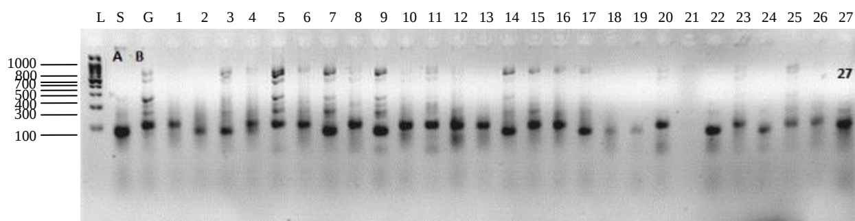
شکل ۱- الگوی نواری محصولاتی PCR تکثیر شده توسط آغازگر RM12091 برای تعدادی از افراد مورد مطالعه. L: پدر، S: والد سپیدرود، G: والد غریب.
