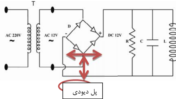
شکل ۲- مدار تشکیل میدان مغناطیسی Figure 2. Circuit formed magnetic field
