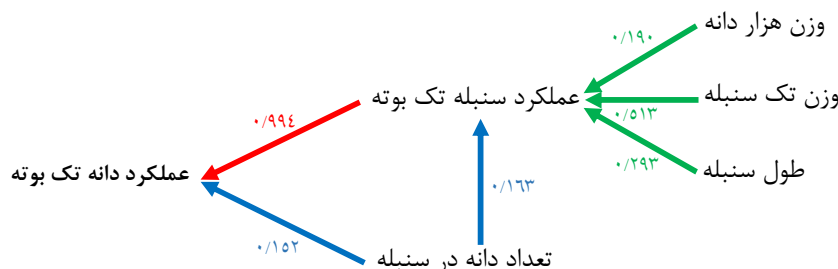
شکل ۱- نمودار تجزیه علیت صفات مؤثر بر عملکرد دانه در شرایط نرمال با حذف اثرات ضعیف Figure 1. The diagram of path analysis of effective traits on grain yield under normal conditions with remove of weak effects
