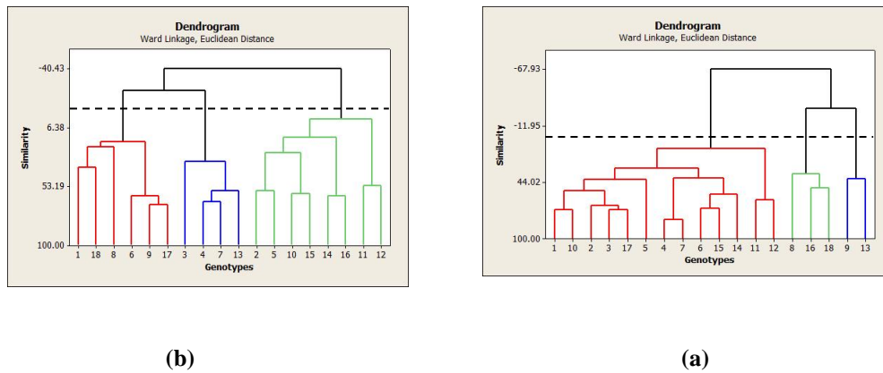
شکل ۱- گروه‌بندی لاین‌های جو مورد استفاده توسط الگوریتم ward و فاصله اقلیدوسی، با استفاده از صفات مورفولوژیک (شکل a) و فیزیولوژیک (شکل b) Figure 1. Grouping of barley lines by Ward algorithm and Euclidean distance using morphological (Fig. a) and physiological (Fig. b) traits
