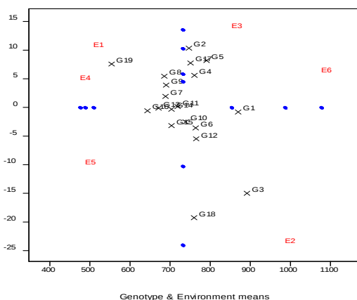
شکل ۱- نمودار بای پلات اثر متقابل ژنوتیپ و محیط بر اساس مولفه اول Figure 1. Genotype and environment interaction biplot based on first component
