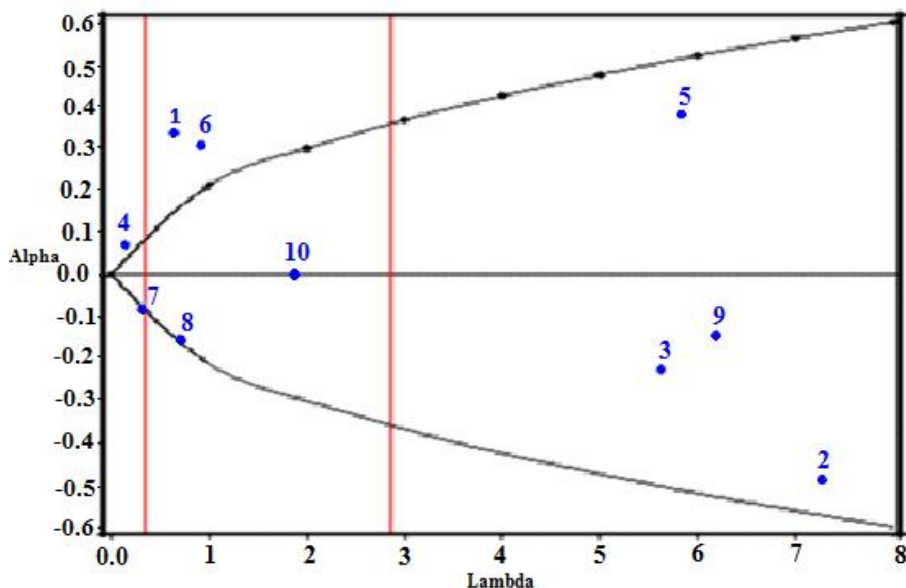
شکل ۲- نمودار برآورد شده با استفاده از رگرسیون تای، برای ارقام آفتابگردان مورد مطالعه (هذلولی فاصله برآورد ۹۵ درصد را برای \alpha = 0 نشان می‌دهد، خطوط عمودی حدود فاصله اطمینان ۹۵ درصد را برای \lambda = 1 نشان می‌دهد).
