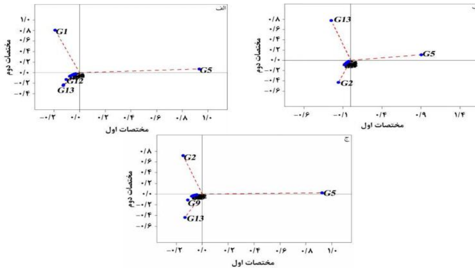
شکل ۱- بای پلات مختصات اصلی اول در مقابل مختصات اصلی دوم با استفاده از روش درخت با حداقل شاخه برای سه سیکل با میانگین کم‌تر از میانگین کل (L).
