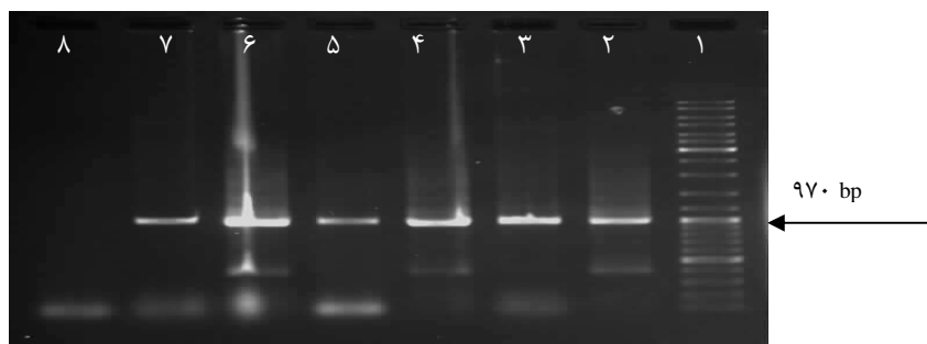
شکل ۲- PCR پلاسمیدهای استخراج شده از کلنی‌های حاصل از واکنش اتصال ناقل pTZ57R/T و پیشبر Pat 1 به منظور بررسی ورود پیشبر Pat 1 و مشاهده باند ۹۷۰ bp (۱) خط کش مولکولی ۱Kbp (۲-۷) محصول PCR حاوی پیشبر pat 1 و مشاهده طول باند ۹۷۰ bp (۸) واکنش PCR آب.
