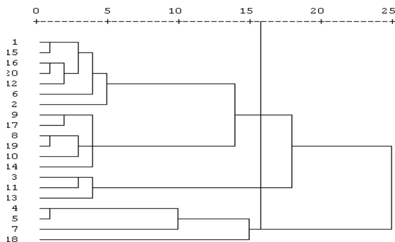
شکل ۳- نمودار درختی حاصل از تجزیه خوشه‌ای به روش حداقل واریانس وارد برای ۲۰ لاین گندم دوروم بر اساس شاخص‌های تحمل خشکی و عملکرد در شرایط دیم و آبیاری تکمیلی
