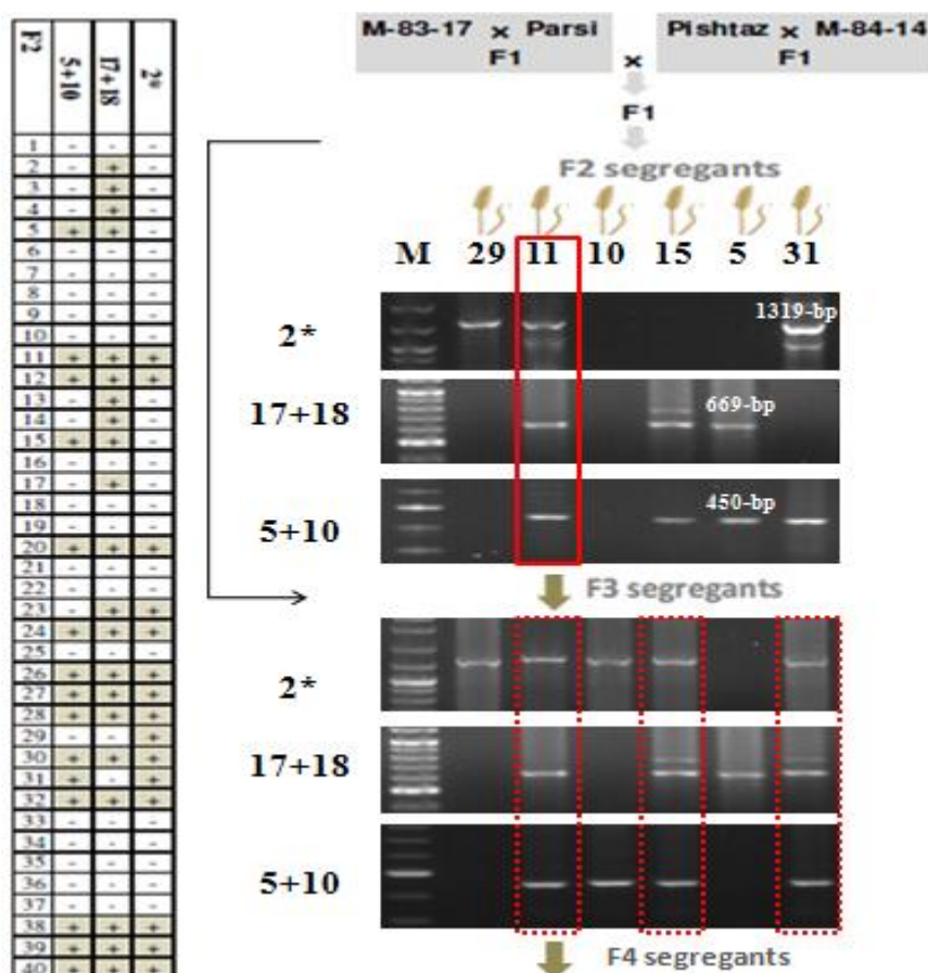
شکل ۲- روند انتخاب نتاج در نسل‌های در حال تفکیک F_2 و F_3 برای بهبود کیفیت نانوائی بر اساس آزمون فعالیت 2^* , Bx17 , Dx5 ، در ۶ نمونه افراد جمعیت F_2 و F_3 گندم هگزاپلوئید تلاقی مربوطه، M: سایز مارکر 100\text{ bp} می‌باشد.
