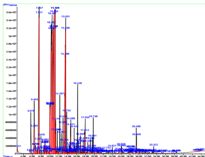
شکل ۱- تصویر کروماتوگرام GC/MS ترکیبات اسانس گیاه نعناع‌فللی در مرحله تمام گلدهی ژنوتیپ همدان Figure 1. The GC/MS chromatogram image of the essential compounds of peppermint plants in the 100%-flowering stage of the Hamadan genotype
