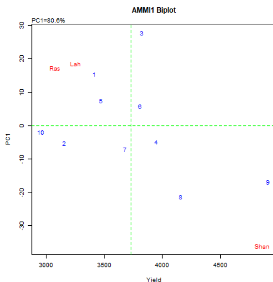
شکل ۱- بای‌پلات میانگین عملکرد غلاف تر لاین‌های پاچ‌باقله، محیط‌ها و مقادیر اولین مؤلفه اصلی آنها (AMMI1) Figure 1. The biplot of mean fresh pod yields of Pachbaghela lines, environments, and values of their first main principal component (AMMI1)
