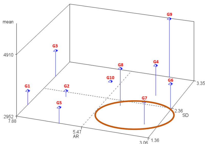
شکل ۳- نمودار سه بعدی عملکرد، میانگین رتبه و انحراف معیار رتبه آماره‌های پایداری لاین‌های پاچ‌باغلا: yield: عملکرد لاین‌های پیشرفته پاچ‌باغلا (کیلوگرم در هکتار). AR: میانگین رتبه‌ها و SD: واریانس رتبه‌ها
