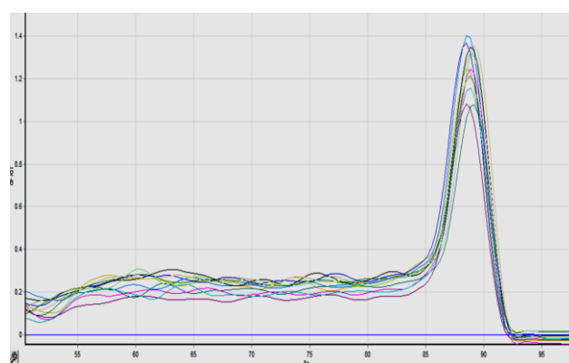
شکل ۳- آنالیز منحنی ذوب PCR Real time ژن کد کننده فارنسیل دی فسفات (FDS) در گیاه درمنه کوهی ( A. absinthium ) Figure 3. Real-time PCR Melting curve analysis of Farnesyl Diphosphate Synthase (FDS) Gene in A. absinthium
