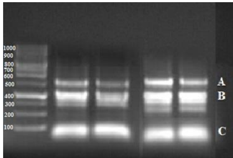
شکل ۲- تصویر الکتروفورز ژل آگارز یک درصد جهت بررسی کیفیت RNA استخراجی نمونه‌های مریم‌گلی ( S. officinalis ) باندها نشان‌دهنده زیر واحدهای (A) 28S rRNA، (B) 18S rRNA و (C) 5S rRNA هستند. اندازه لدر 100 bp است.
