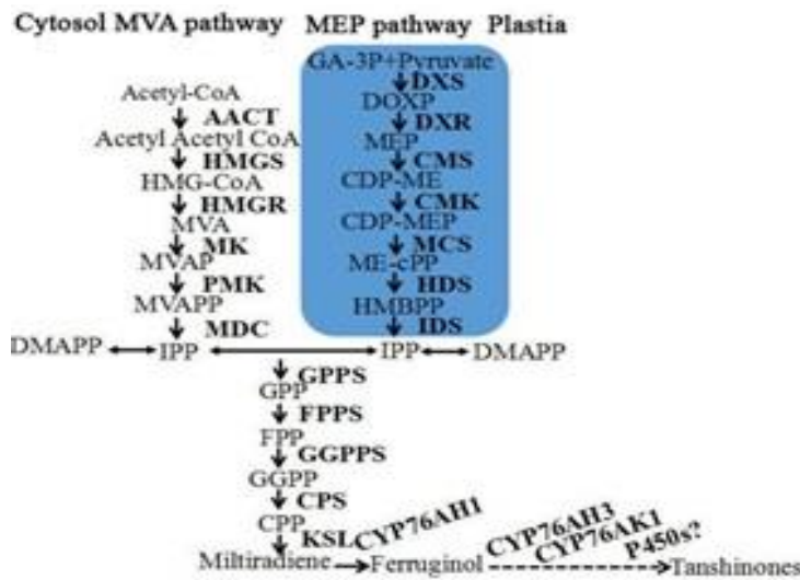
شکل ۱- مسیر سنتز تانشینون‌ها در گیاهان (۳۷) Figure 1. The biosynthesis pathway of tanshinones in plants (37)
